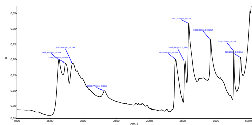
Рис.1. ИК-спектр тиомочевины
